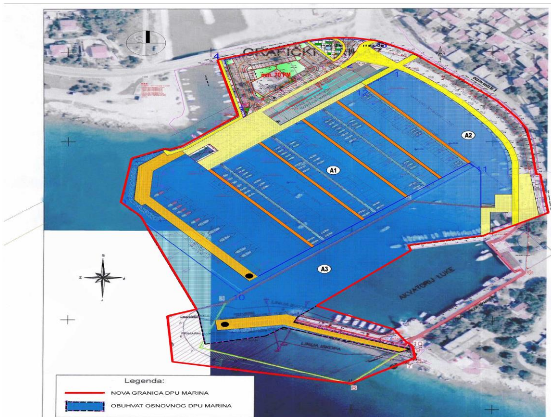
Luka Novi – predviđena dogradnja primarnog i sekundarnog lukobrana u sklopu marine
