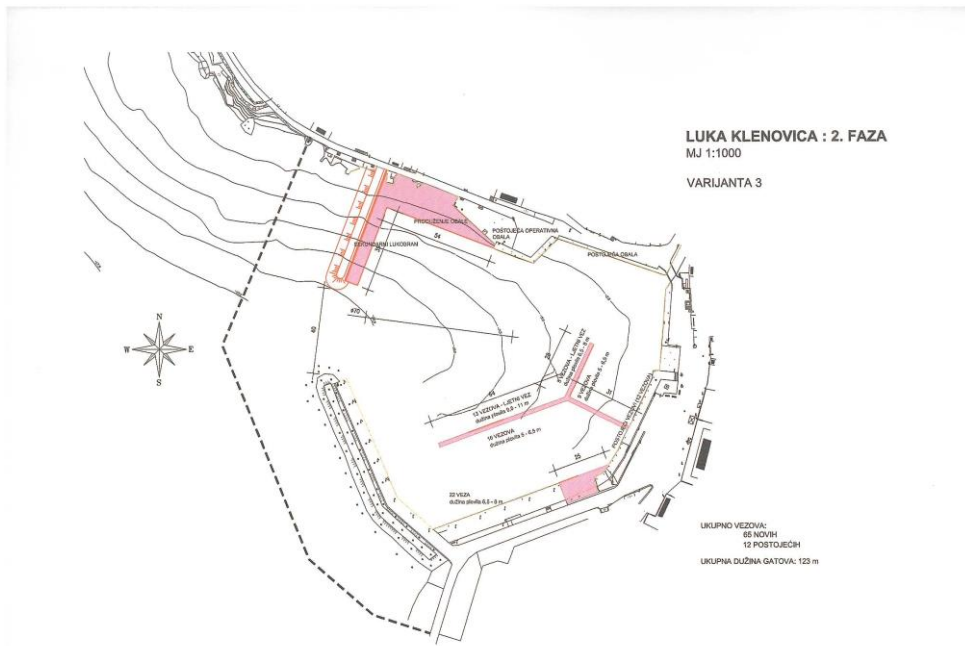
II. faza ribarske luke Klenovica- izgradnja sekundarnog lukobrana i gatova
