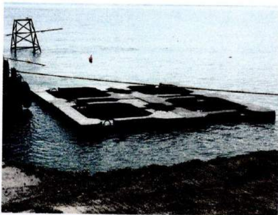
Radovi – izgradnja sekundarnog lukobrana
