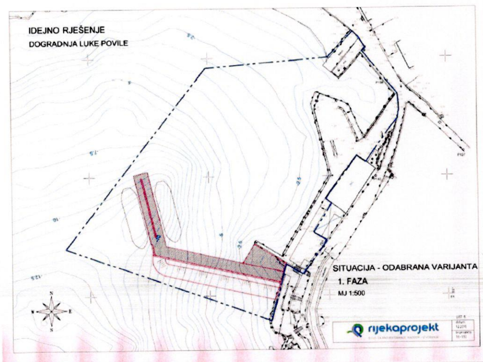
Izgradnja lukobrana i obale – luka Povile
